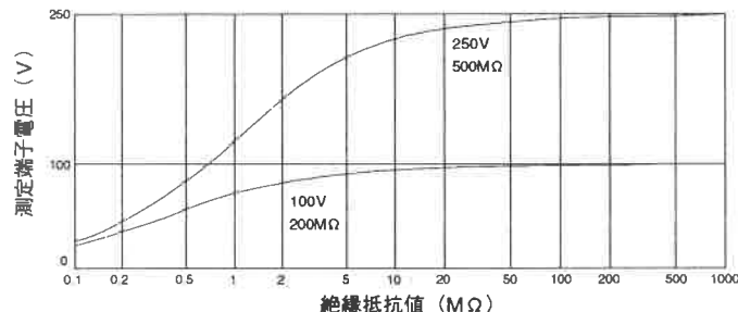
図1. SK-3000 電圧特性
